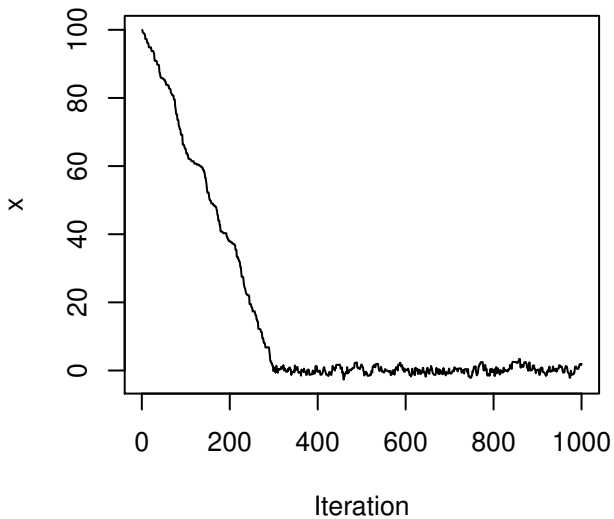
RWM x_0=100
