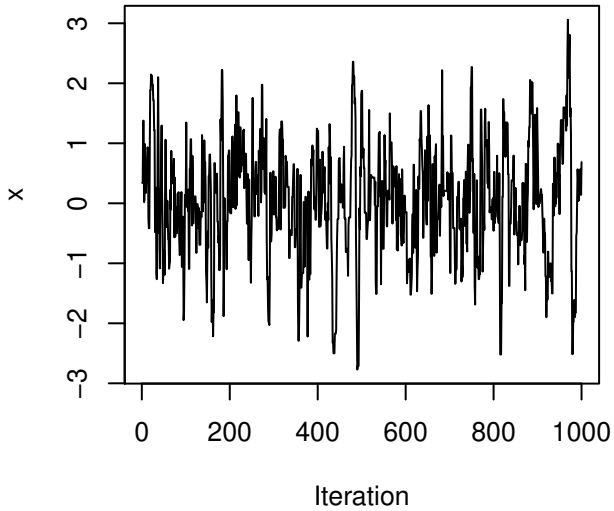
RWM - N(0,1)
