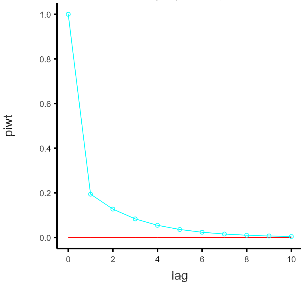
ARMA(1,1) model piwt
