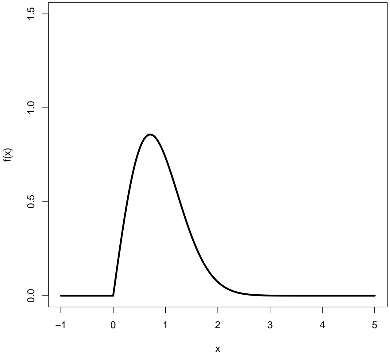
Weib(2,1)
